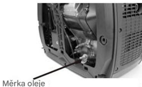
Obrázek 2 – Otvor pro plnění oleje, měrka a hladina oleje
