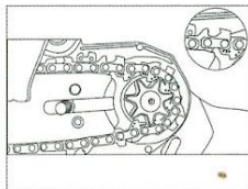
3. Umístěte řetěz kolem řetězového kola a ujistěte se, že vodící lišta je zarovnána s čepem. Upozornění!!! Řetězová pila musí být nainstalována ve správném směru.
